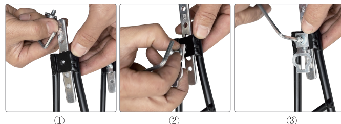
① ② ③ Nastavení výšky nosiče | Adjust the carrier height
